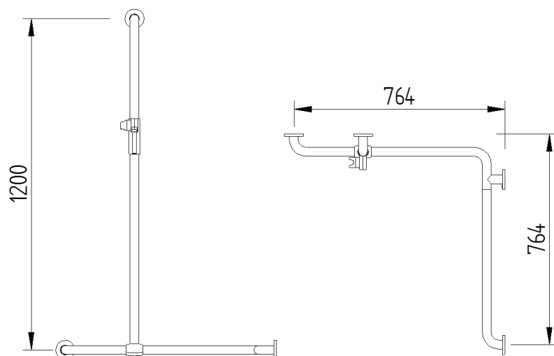
Technische Zeichnung (Ausführung Links)
