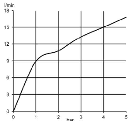
Durchflussdiagramm
