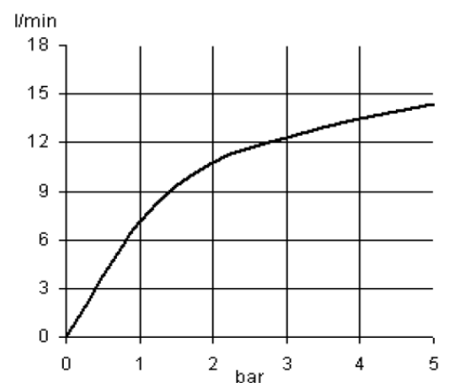
Durchflussdiagramm
