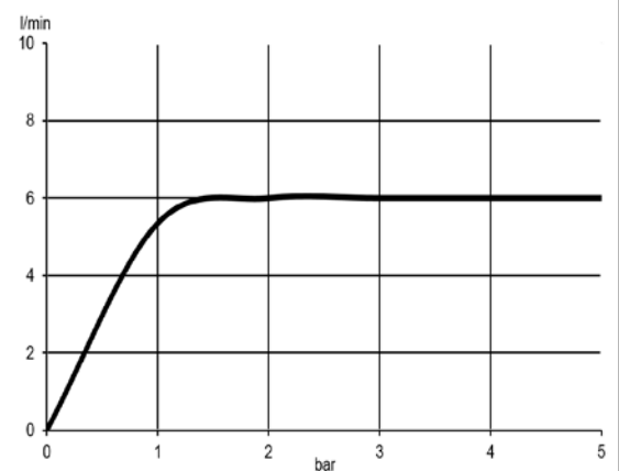
Durchflussdiagramm
