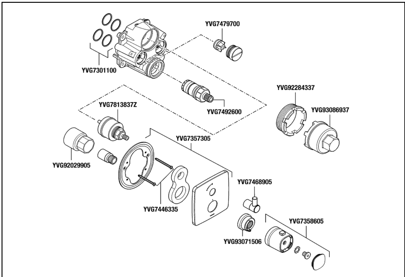
WHITENFTM Farbset Thermostat white für VIGOUR -Box VIGUPK mit Mengenregulierung verchr.VIGOUR Thermostat finish set white for VIG. Box VIGUPK with volume regulator chr.VIGOUR
