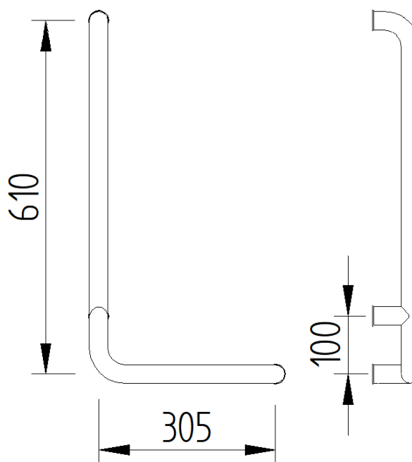
Technische Zeichnung (Ausführung Links)
