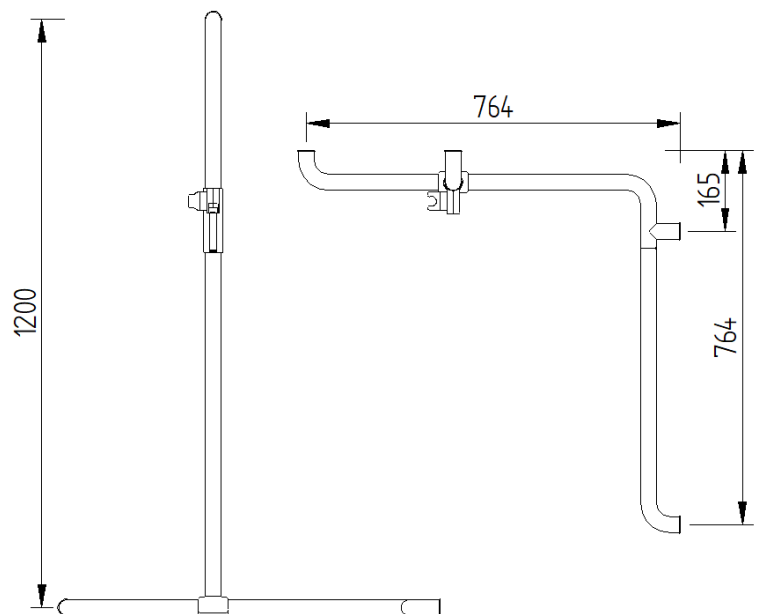
Technische Zeichnung (Ausführung Links)
