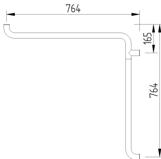
Technische Zeichnung (Ausführung Links)
