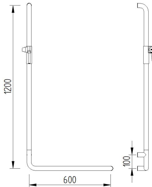
Technische Zeichnung (Ausführung Links)
