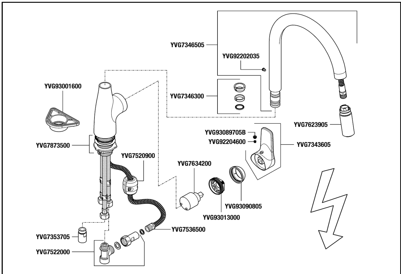
DESPNDUAA Einhand-ND-Spültischbatterie derby mit herausz. U-Auslauf schwenkb. verchr. VIG Single lever LP sink mixer Derby extricable U-spout slewable chr. VIGOUR
