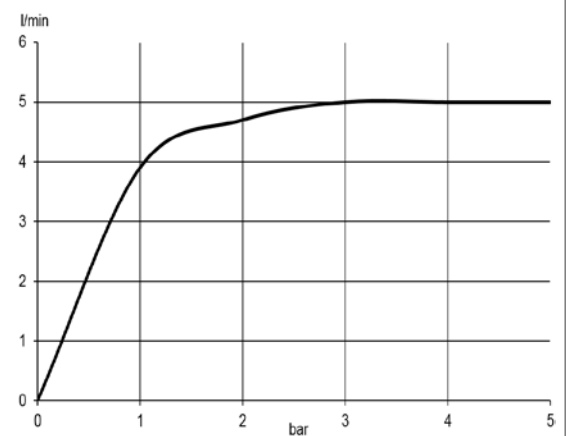
Durchflussdiagramm
