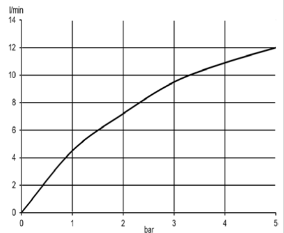
Durchflussdiagramm
