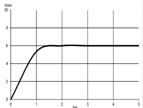
Durchflussdiagramm
