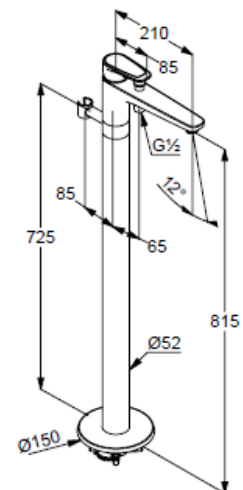
Maßzeichnung
