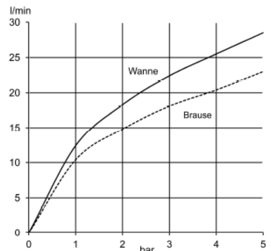
Durchflussdiagramm
