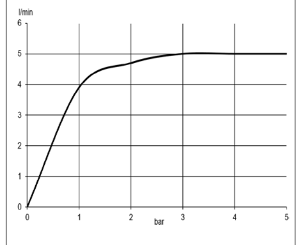
Durchflussdiagramm
