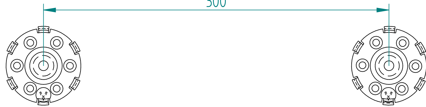
Montageskizze
