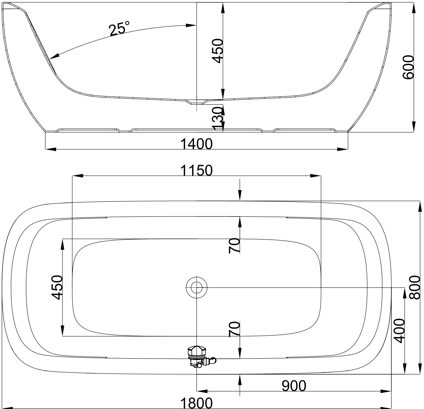
Mittelablaufwanne Acryl Derby 1800 x 800 Monoblock freistehend mit Überlaufbefüllung Art.-Nr.463401 / Vigour Art.Nr. DEAMF180UBV Alle Maßangaben in mm. Technische Änderungen vorbehalten
