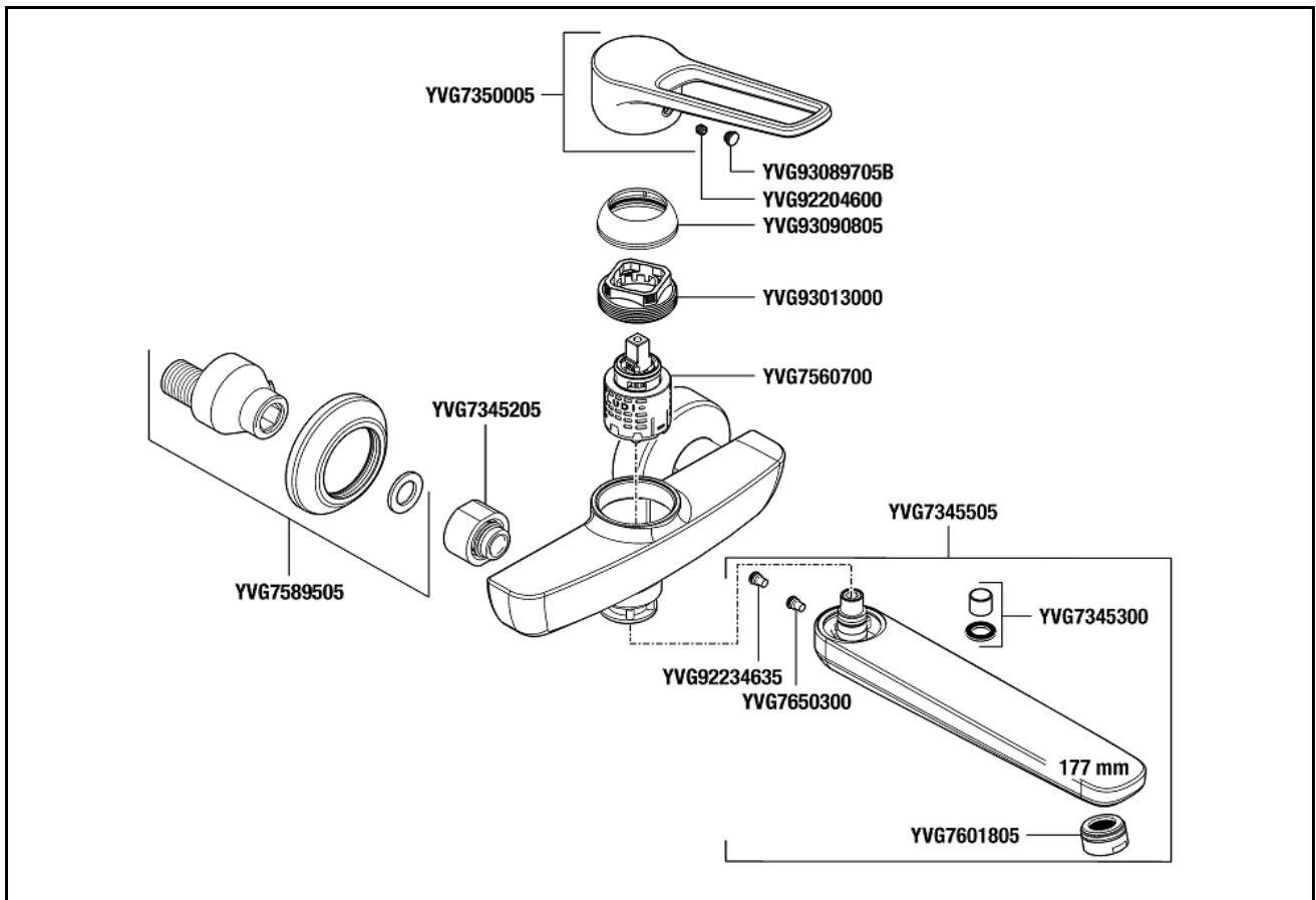
DEPOHWB245 Einhand-Wandbatterie derby plus m. Hebel offen Ausl. 245mm m.absp.S-Anschl.vc VIG
