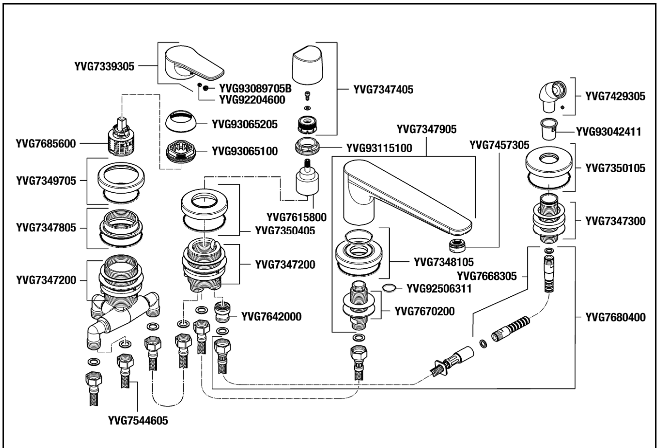
DEFL4 Vierloch-Badebatterie derby 4-hole bath mixer derby mit Auslauf 220mm o. Handbrause VIGOUR Spout 220mm without Handshower VIGOUR
